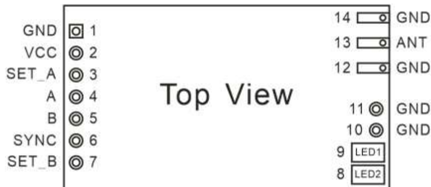
VT-SA04C 尺寸图 38.0 × 21.4mm, 数据接口引脚间距 2.54mm
